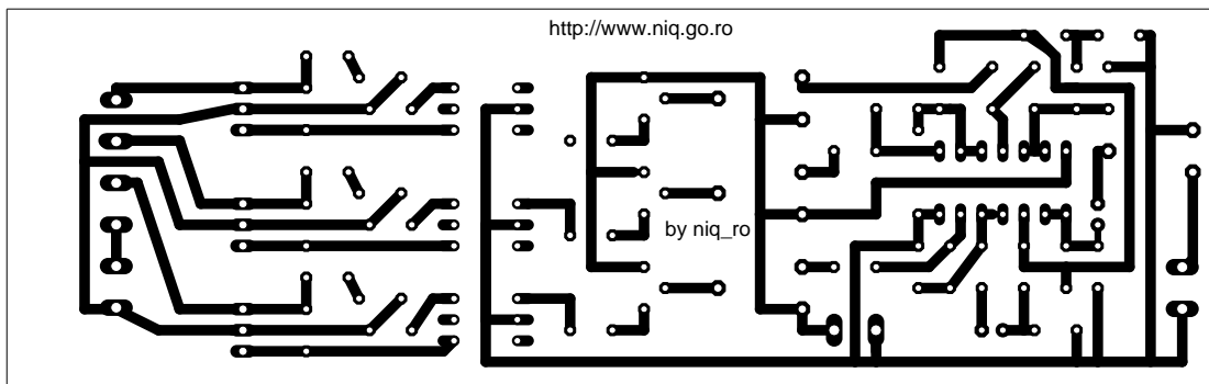
orga de lumini schema originala Tehnium 7/88 + adaugare optocuploare
